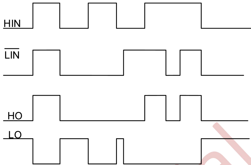
图 9-1 G2022 输入输出时序波形
